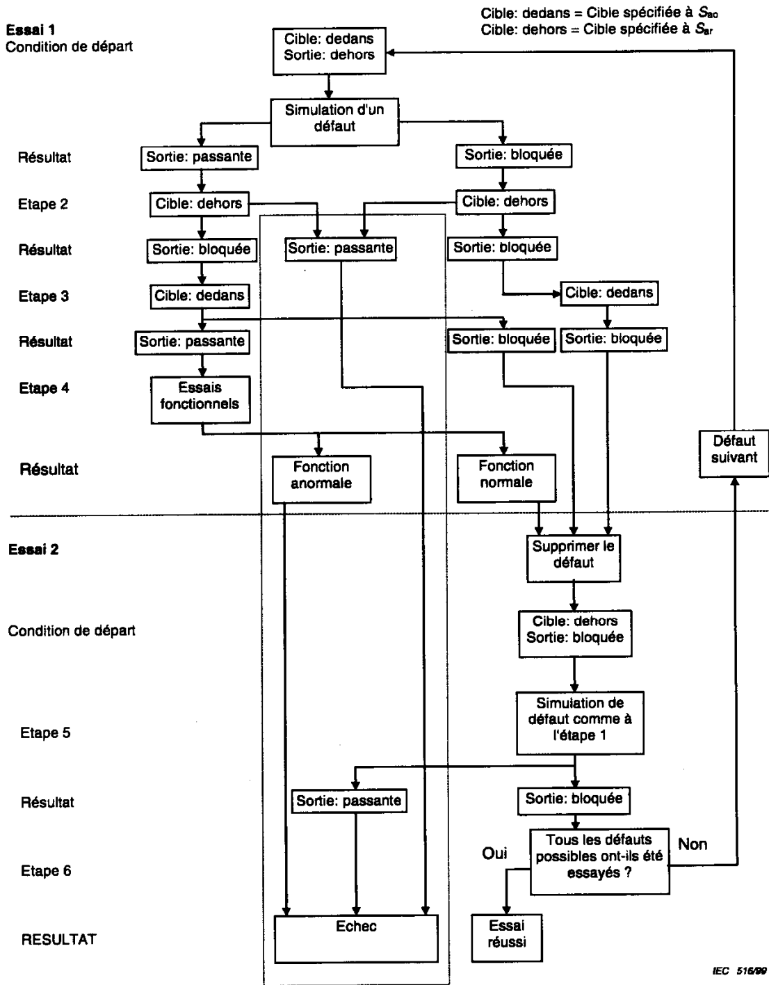
Figure A.2 – Séquence d'essais pour PDF-S
