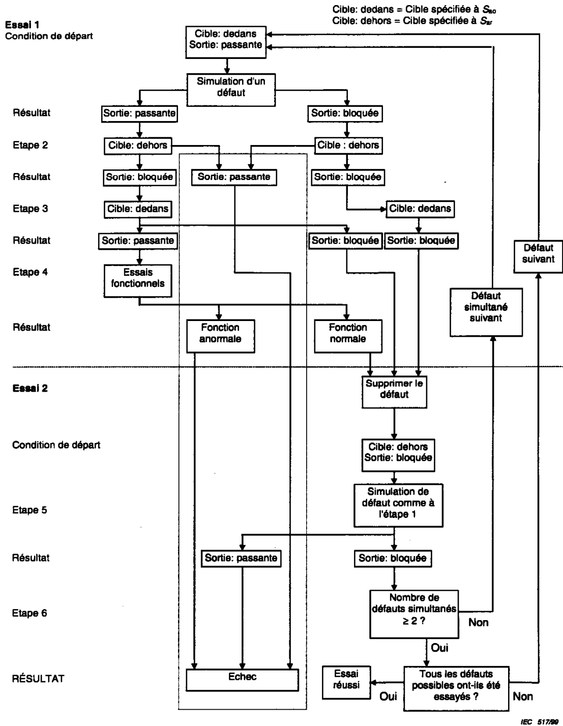
Figure A.3 – Séquence d'essais pour PDF-M
